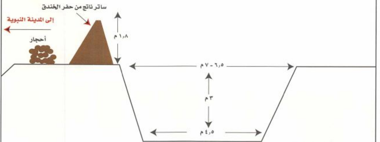
الأبعاد التقريبية للخندق
